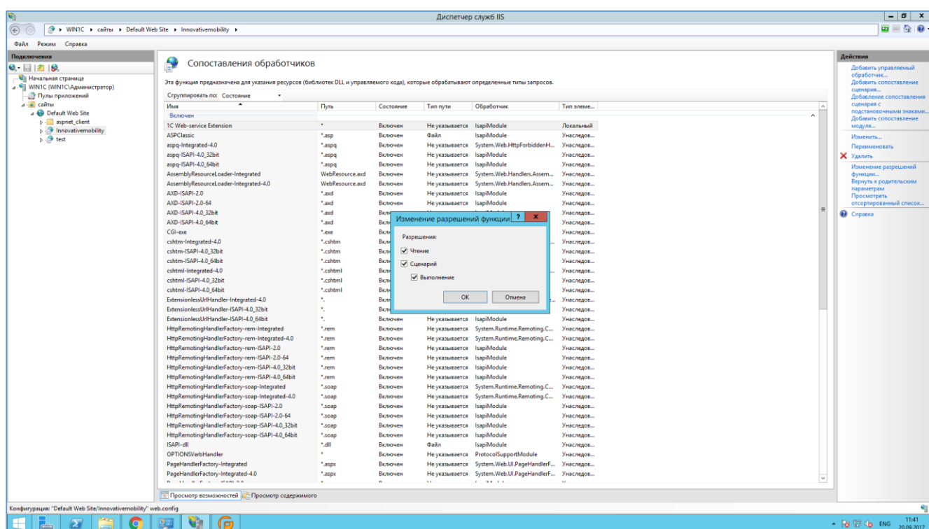
Рисунок 17 – Запрет на вход пользователя import_user в базу 1С
