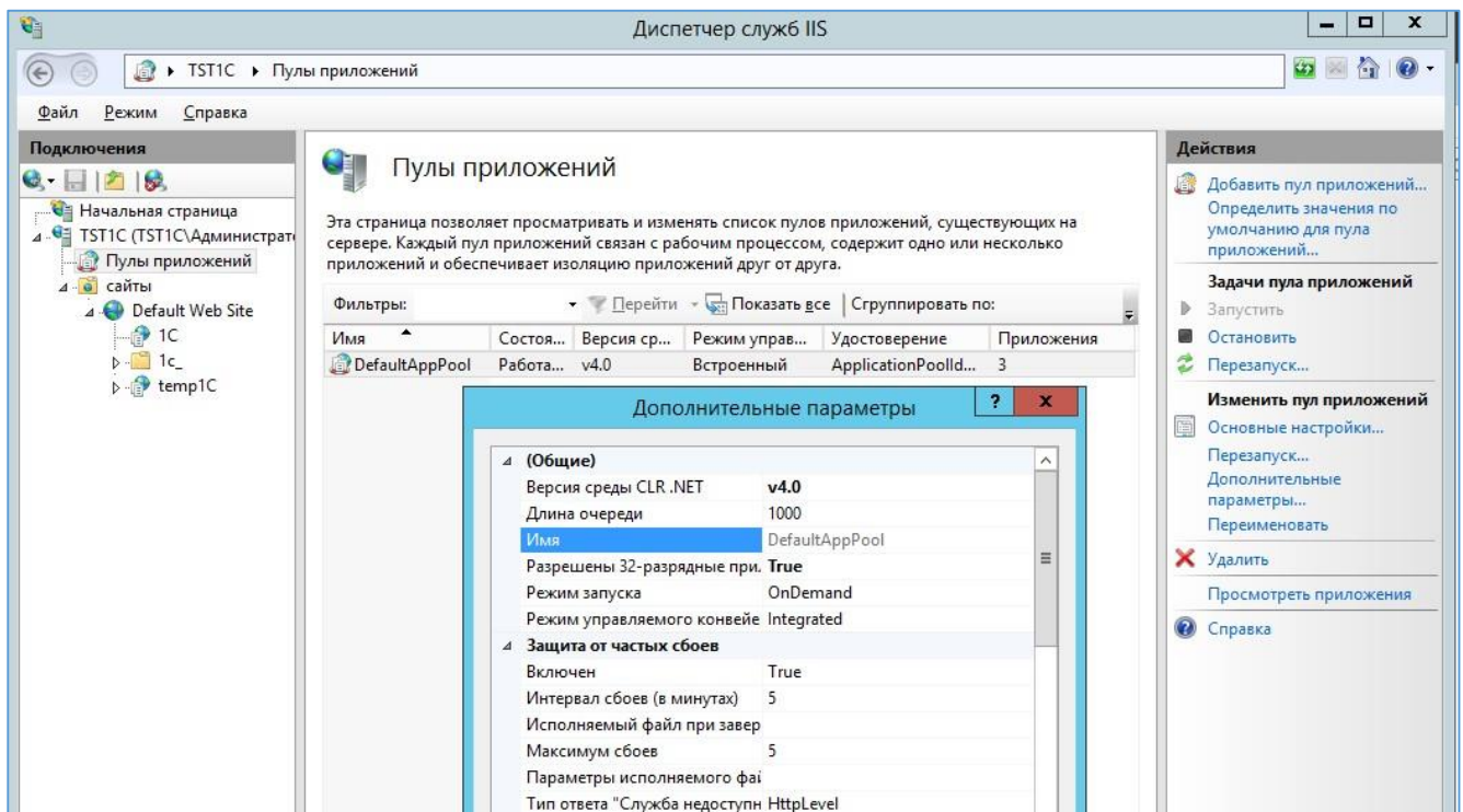
Рисунок 30 – Изменение режима для обработчика
