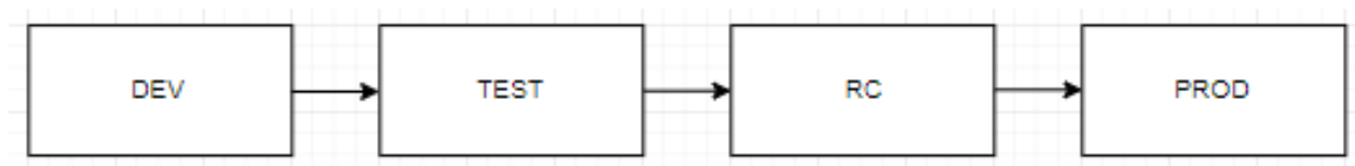
Рисунок 7 – Этапы тестирования
