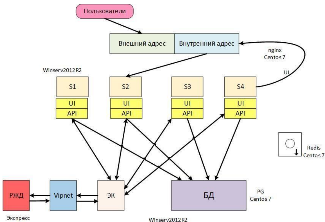
Рисунок 1 – Общий вид системы
